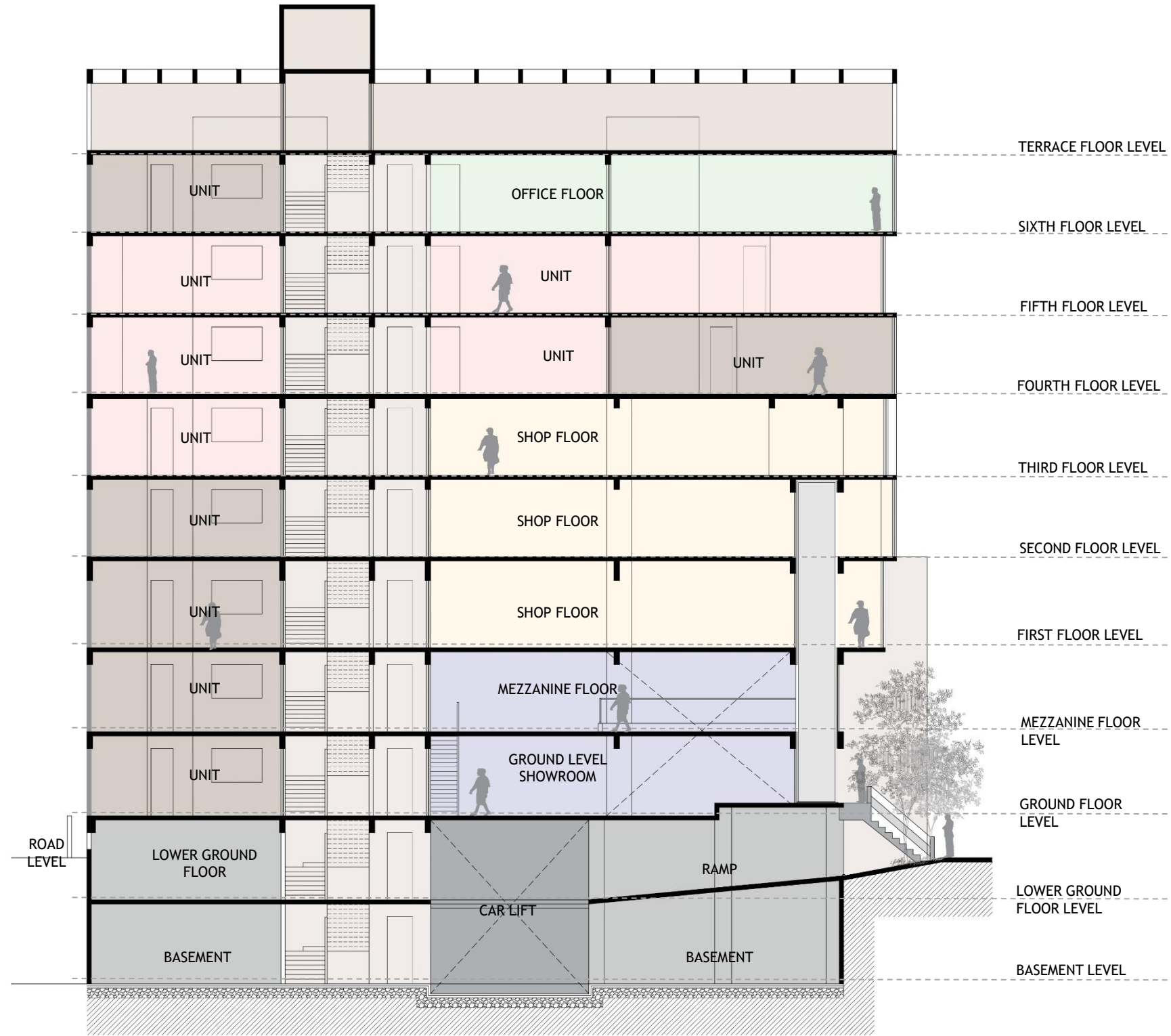
Section A-A'
